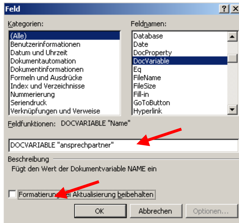
Abbildung 7: Feldbenennung
