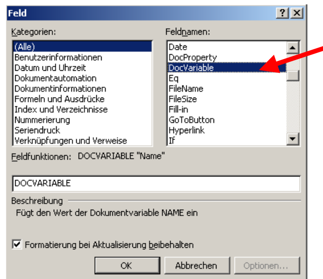
Abbildung 6: Dialog Feldeinfügen
